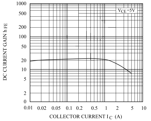
h_{FE} - I_C
