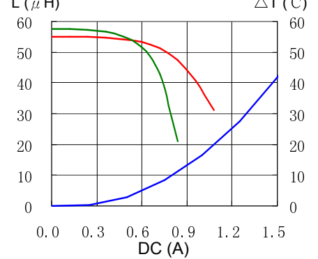
18. CDRH6D38NP-101NC
