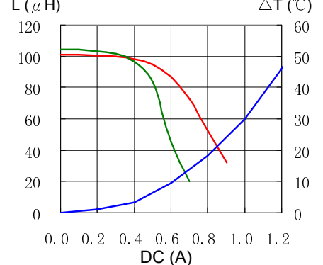
18. CDRH6D38NP-101NC
