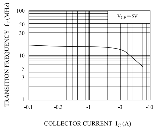
f_T - I_C
