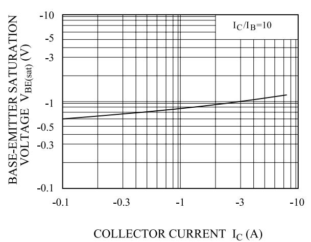
V_{BE(sat)} - I_C
