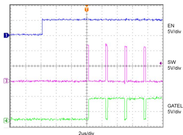
Figure 28: Enable (EN) Delay, 0A
