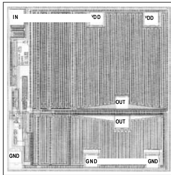
DIE SIZE 76x77 (mm)
