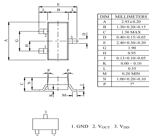
SOT-23
