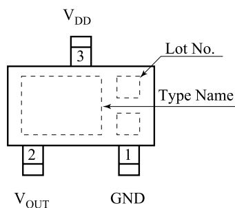
SOT-23
