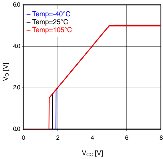
Fig. 27 V CC -V O (I O =0mA)
