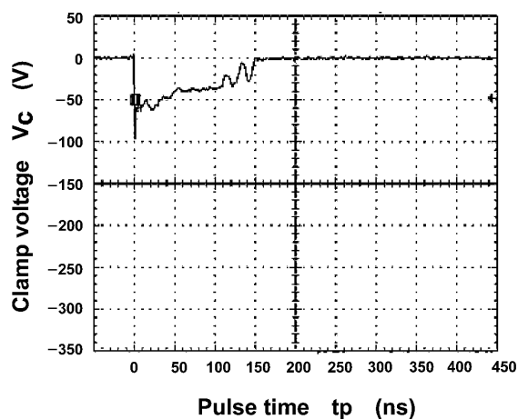
Fig. 10.2 -8 kV
