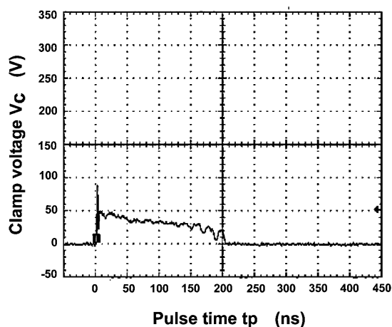
Fig. 10.1 +8 kV
