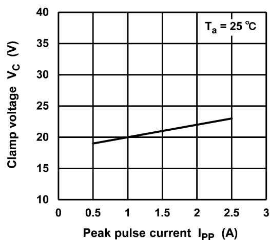
Fig. 9.1 V_C - I_{PP}
