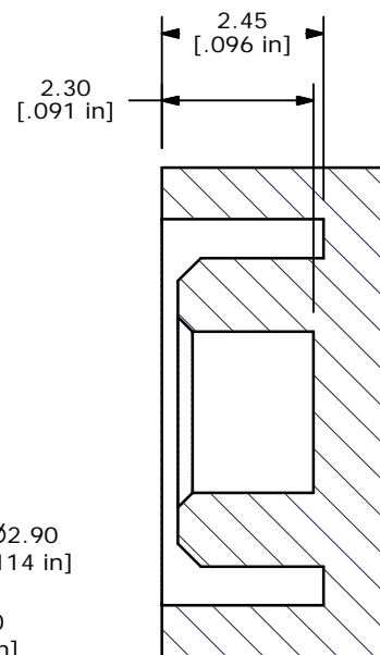
SECTION A-A SCALE 8 : 1
