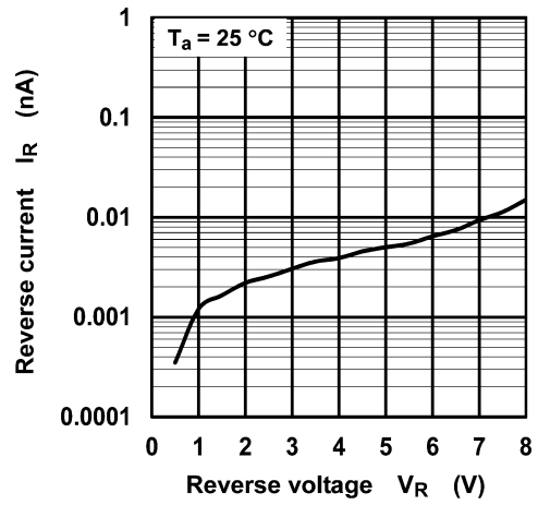
Fig. 8.2 I_R - V_R
