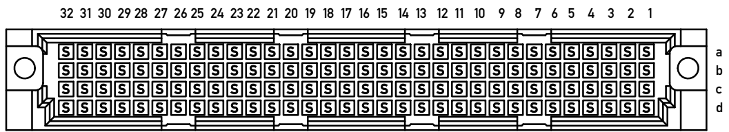
Leiterplatten-Lochbild / PCB drillhole pattern
