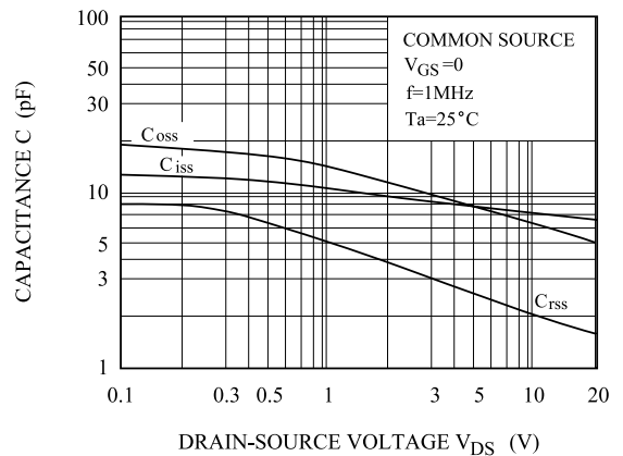
C - V_{DS}
