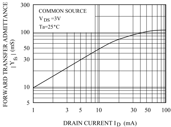
|Y_{fs}| - I_D
