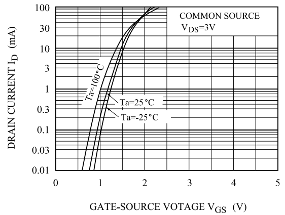
I_D - V_{GS}
