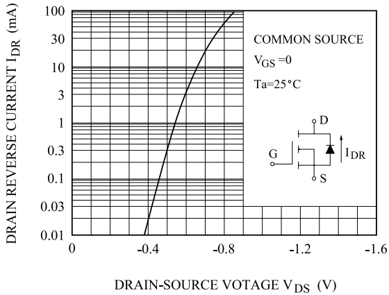
I_{DR} - V_{DS}
