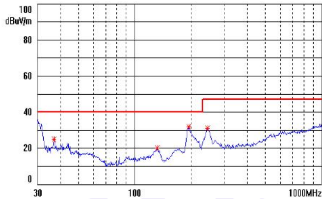
URA4815LD-20WR2 RE(Horizontal)
