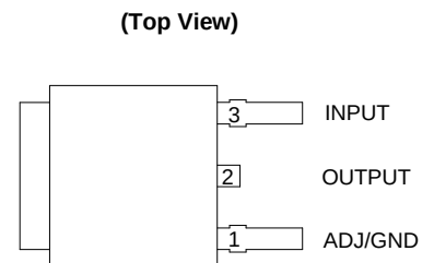
TO252-2 (5)
