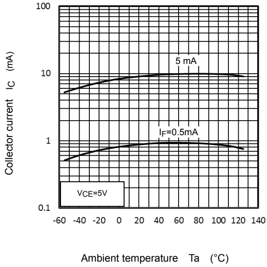
I_C - T_a
