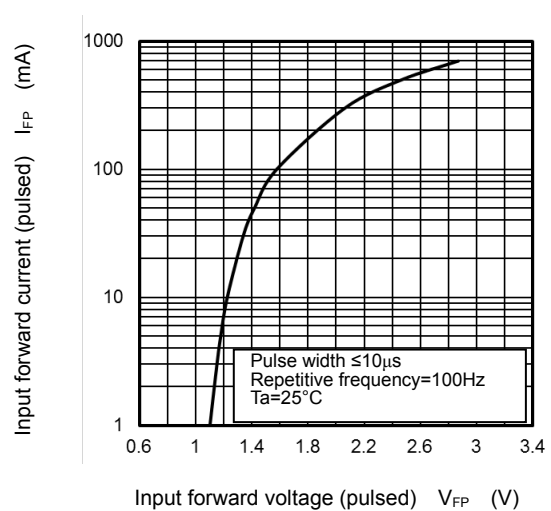
I_{FP} - V_{FP}
