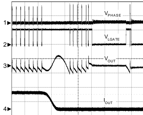
Load Transient 10A->0A
