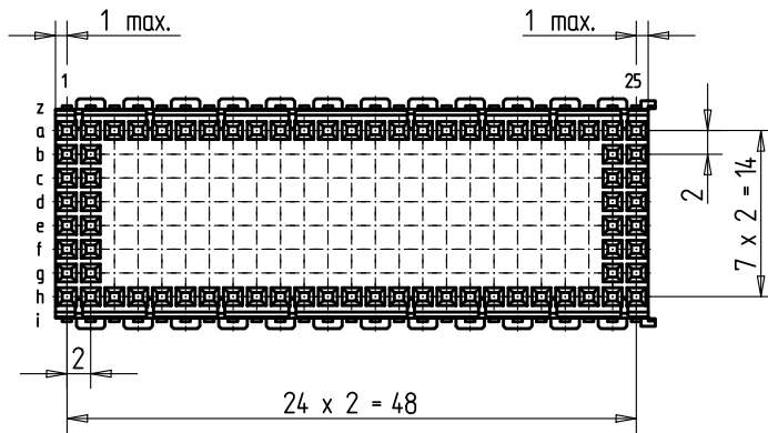
Bestückungsplan - contact layout
