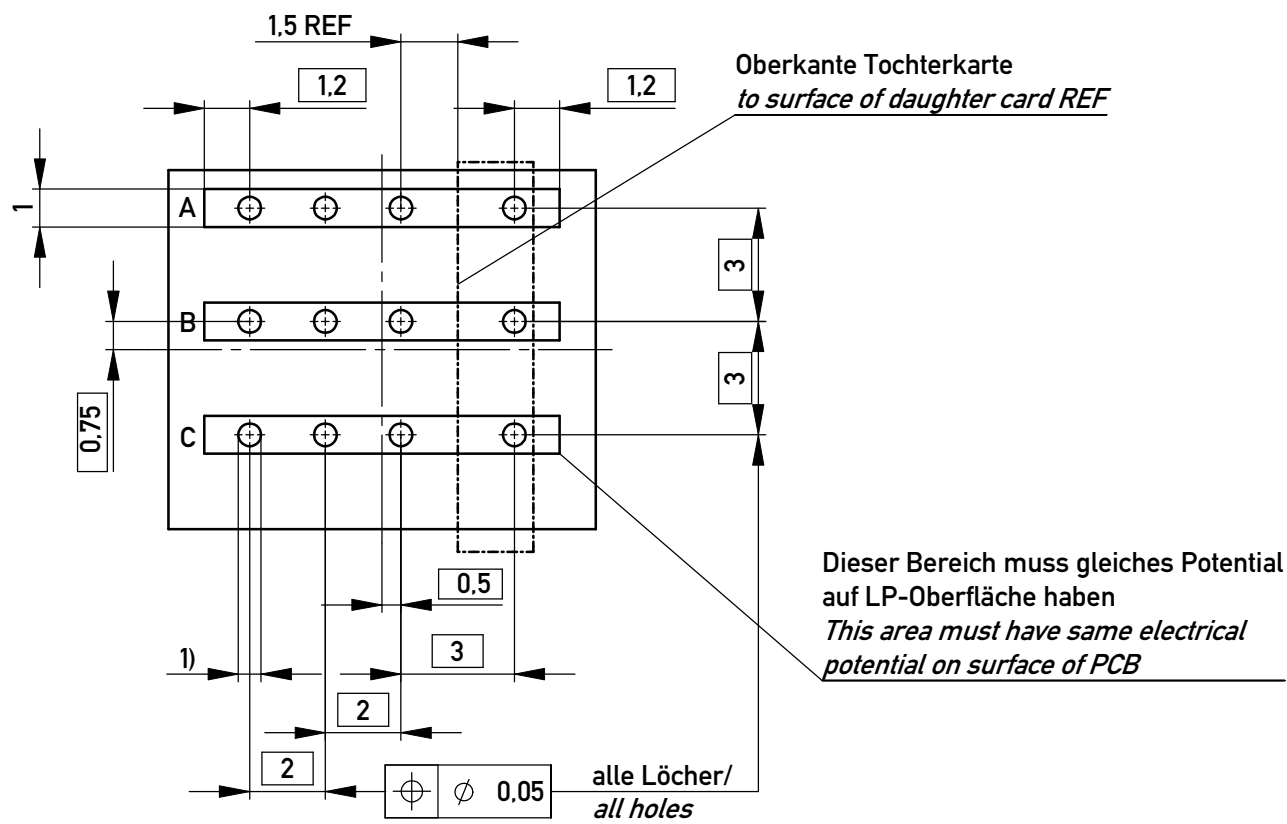
Lochbild für Leiterplatte / Board hole pattern
