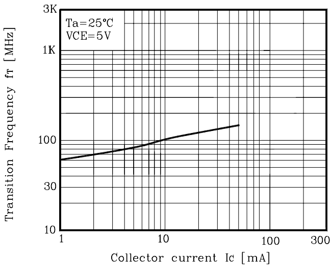
Fig. 11 f_T - I_C
