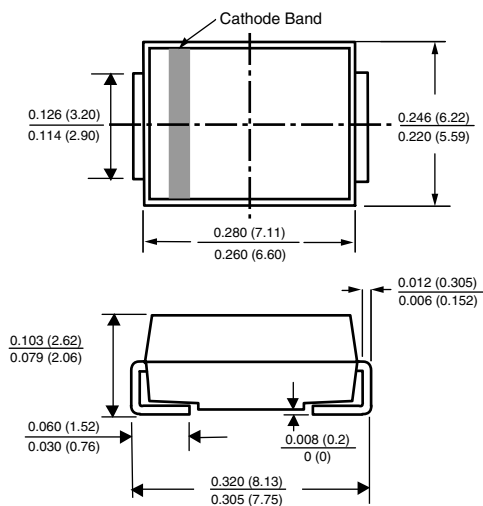
DO-214AB (SMC)
