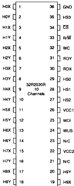
36-Pin SOM
