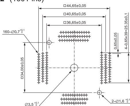
QFP IC234-1764-005 (176 Pins)
