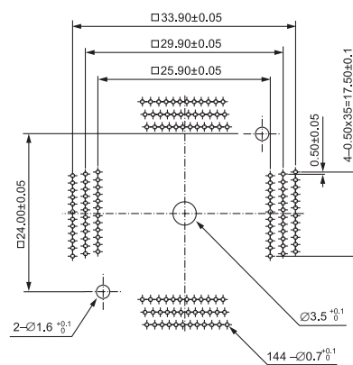
QFP IC234-1444-016 (144 Pins)
