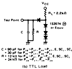
(b) TTL Load
