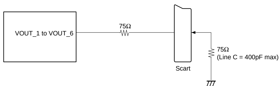
Fig. 16. Video Output Interface
