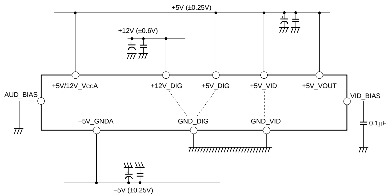
Fig. 24. Dual Supply
