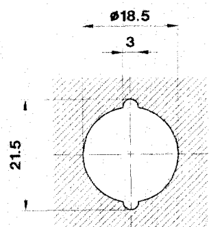
Bohrplan Drilling plan Plan de perçage
