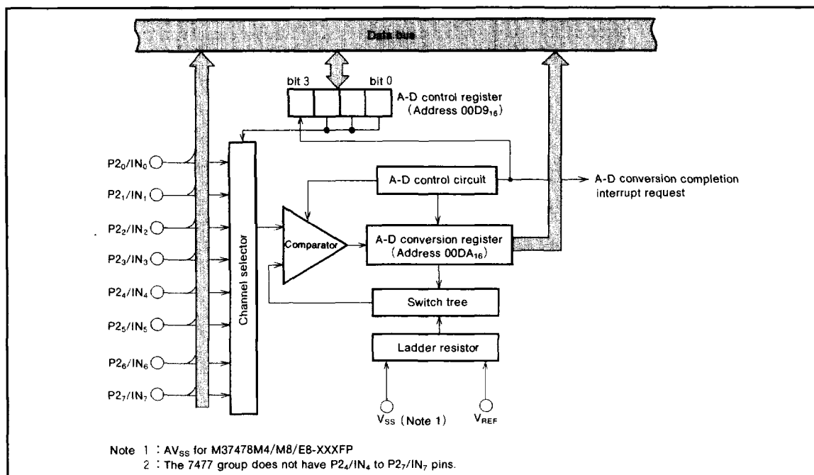
Fig. 13 A-D converter circuit
