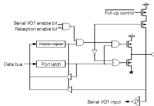
(8) Port P46
