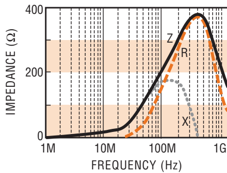
FBM0603-241 □
