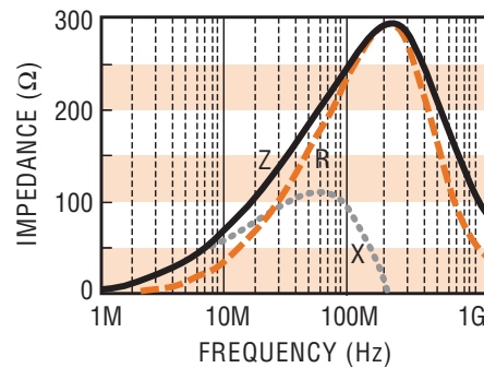
FBM0805-241 □
