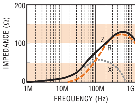
FBM0603-800 □
