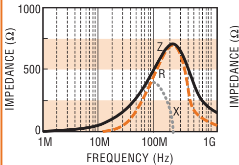
FBM0603-471 □
