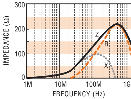
FBM0603-121 □
