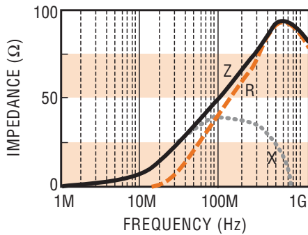
FBM0603-600 □
