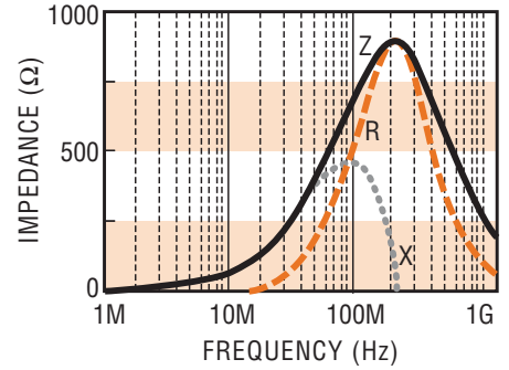
FBM0603-102 □
