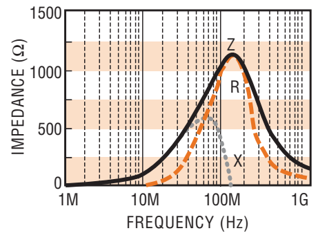
FBM0603-152 □
