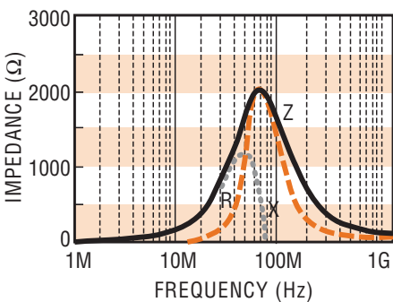
FBM0805-202 □
