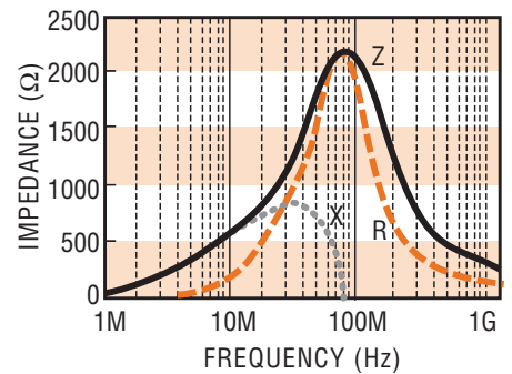
FBM0603-202 □
