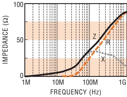
FBM0603-400 □
