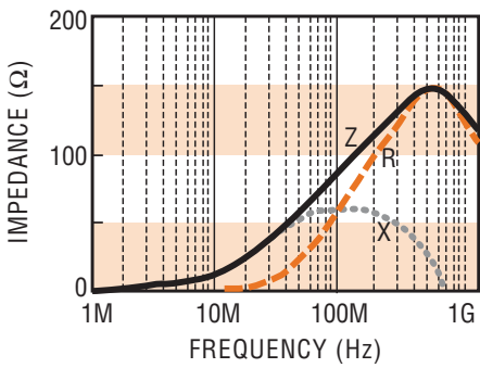
FBM0805-800 □
