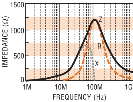
FBM0805-102 □
