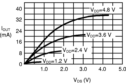
V_{DS} - I_{OUT}
