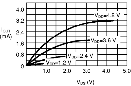
V_{DS} - I_{OUT}
