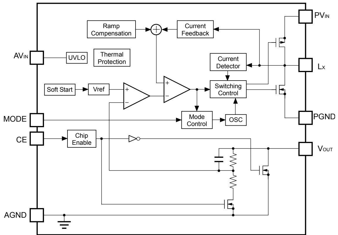
RP505K001C
