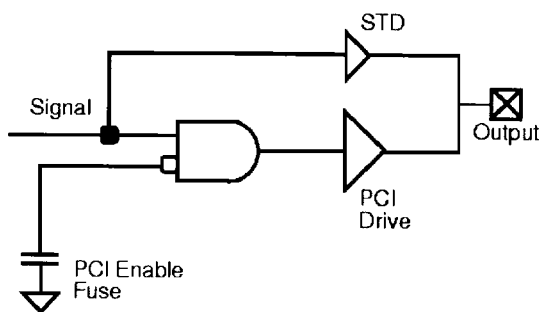
Figure 6• I/O Module
