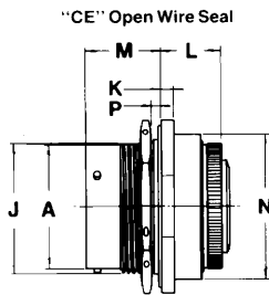
PT07CE-XX-XXX SP07CE-XX-XXX
