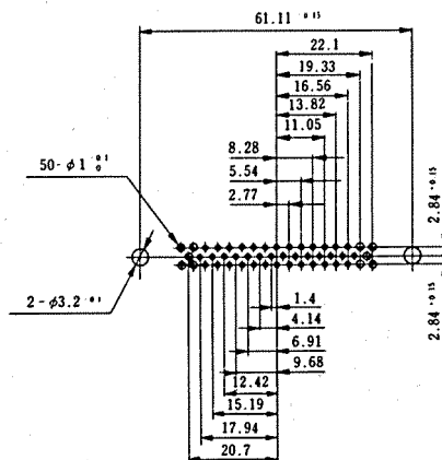
SDBB-25
