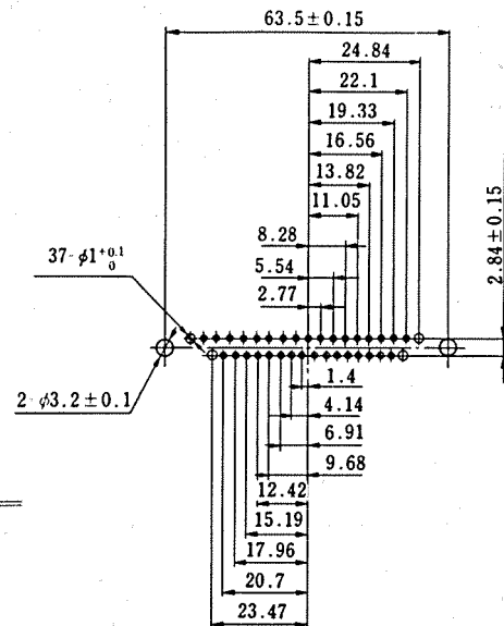
SDCB-37
