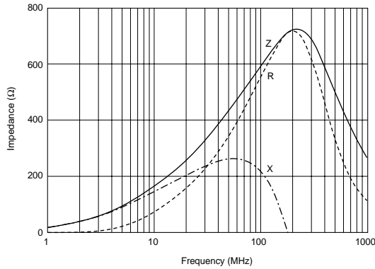
BLM18AG601SN1
