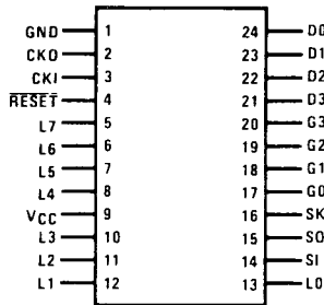
Order Number ET 9421/N, ET 9321/N Package N24A
