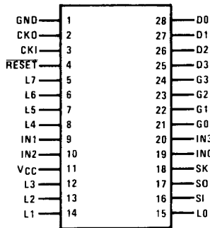
Order Number ET 9420/N ET 9320/N Package N28A
