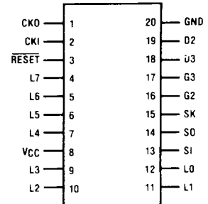
Order Number ET 9422/N ET 9322/N Package N20A
