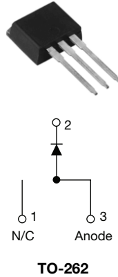
VS-MURB1520-1PbF
