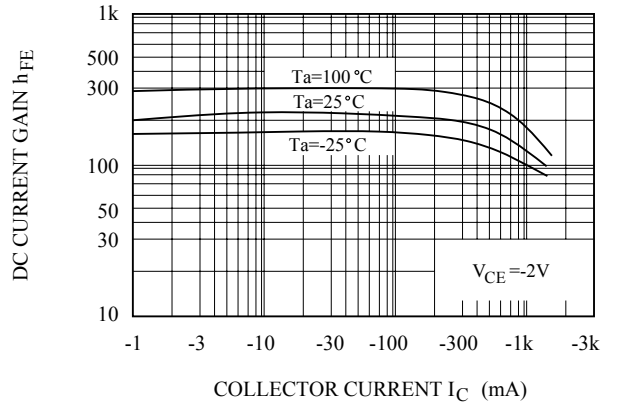
h_{FE} - I_C
