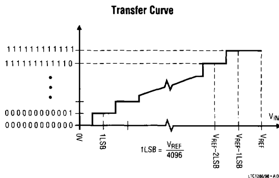
Output Code
