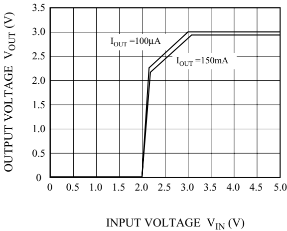
Fig. 3 V_{IN} - V_{OUT}
