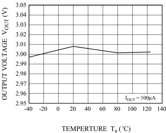
Fig. 5 T_a - V_{OUT}
