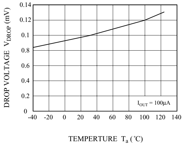
Fig. 4 T_a - V_{DROP}
