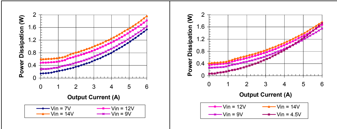
V_o = 5V
