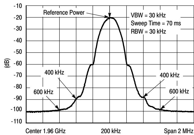
Figure 14. EDGE Spectrum
