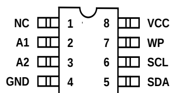
8 pin SOIC
