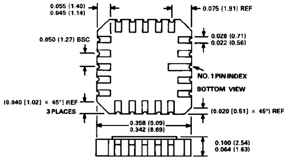
20-Pin LCC
