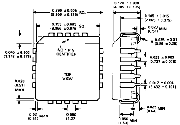
20-Pin PLCC
