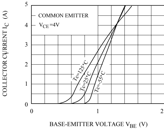
I_C - V_{BE}
