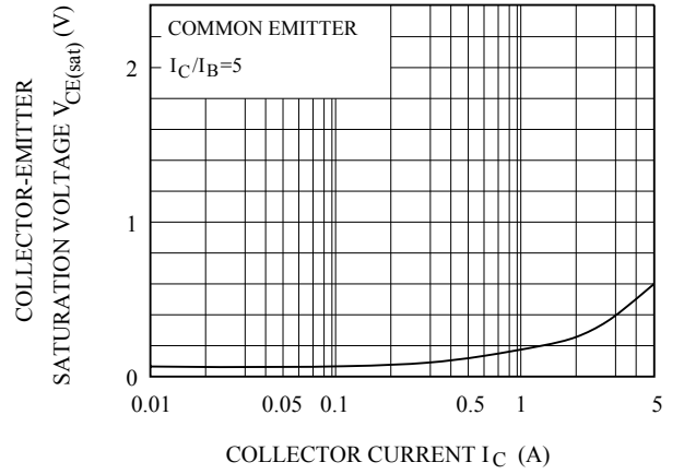
V_{CE(sat)} - I_C
