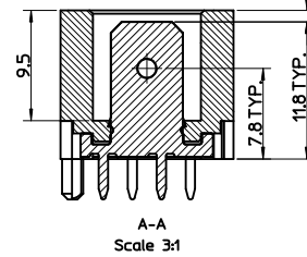
A-A Scale 3:1
