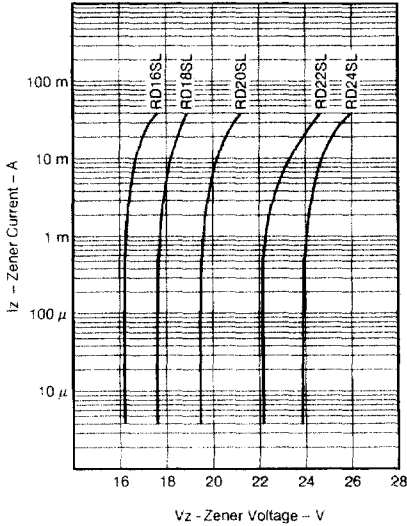
Fig. 4 ZENER CURRENT vs. ZENER VOLTAGE
