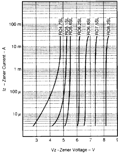
Fig.2 ZENER CURRENT vs. ZENER VOLTAGE
