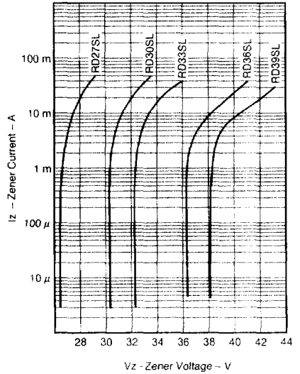
Fig. 5 ZENER CURRENT vs. ZENER VOLTAGE
