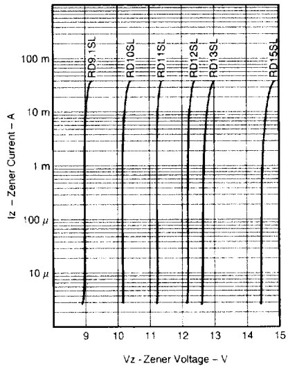
Fig. 3 ZENER CURRENT vs. ZENER VOLTAGE
