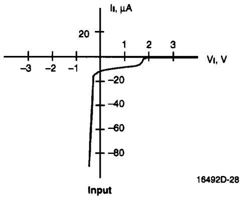
Input
