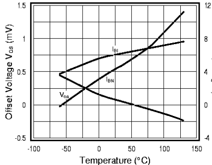
I_{B1} , I_{B2} , V_{OS} vs. Temperature
