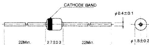
DO-34 (MSD)
