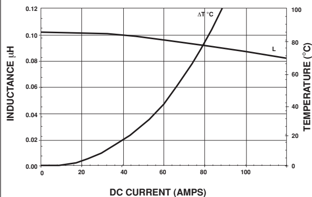
IHLP-5050EZ-01 0.10 \mu H
