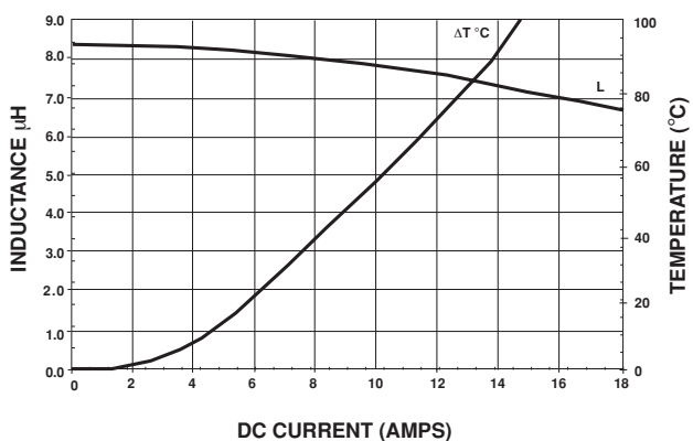
IHLP-5050EZ-01 8.2 \mu H
