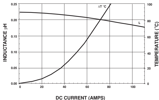
IHLP-5050EZ-01 0.22 \mu H
