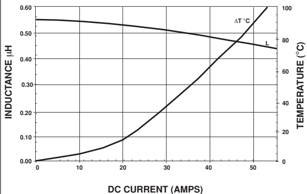
IHLP-5050EZ-01 0.56 \mu H
