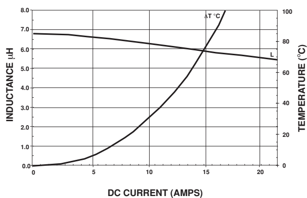
IHLP-5050EZ-01 6.8 \mu H
