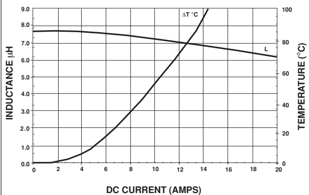
IHLP-5050EZ-01 7.8 \mu H
