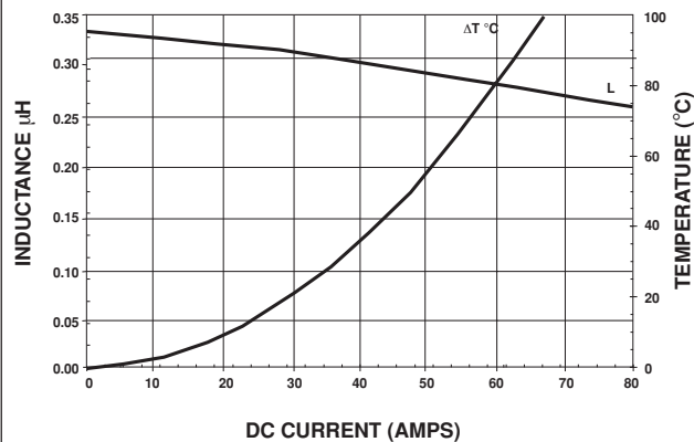
IHLP-5050EZ-01 0.33 \mu H
