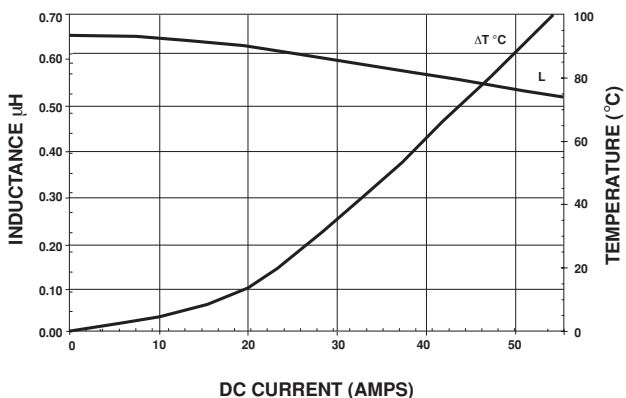
IHLP-5050EZ-01 0.68 \mu H
