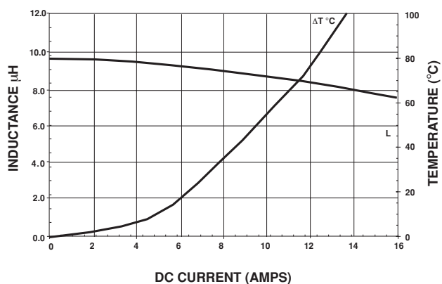
IHLP-5050EZ-01 10 \mu H
