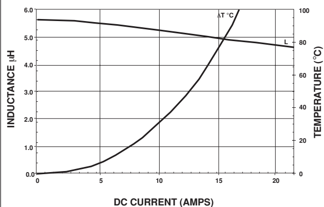
IHLP-5050EZ-01 5.6 \mu H
